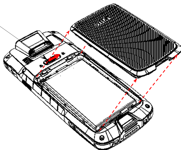
Рисунок 5. Отделение крышки отсека для АКБ от корпуса
