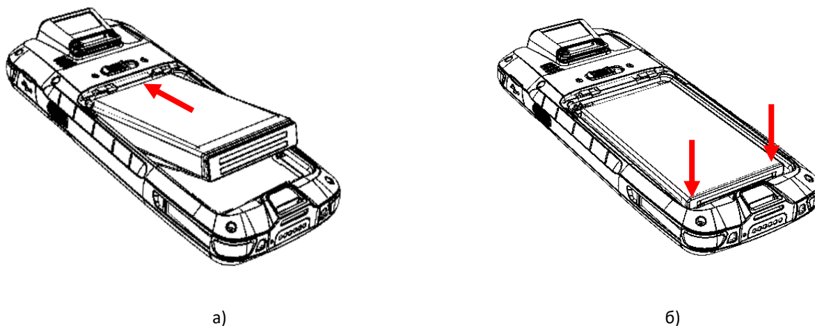
Рисунок 7. Установка АКБ: а) совместить контакты АКБ и блока управления ТСД; б) надавить на нижнюю часть АКБ.
