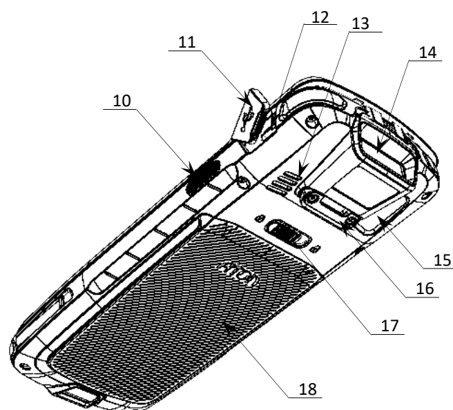
Рисунок 2. Вид сзади/справа
