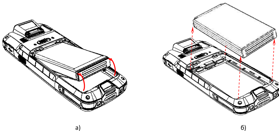
Рисунок 6. Извлечение аккумулятора: а) отделить нижнюю часть АКБ; б) извлечь АКБ
