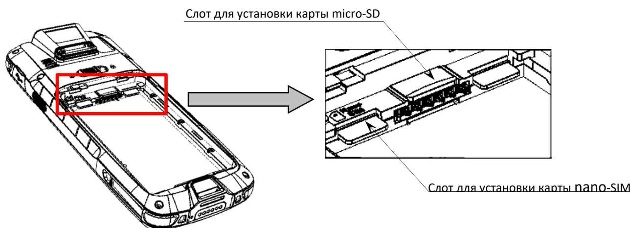
Рисунок 8. Расположение слотов для карт nano-SIM и micro-SD
